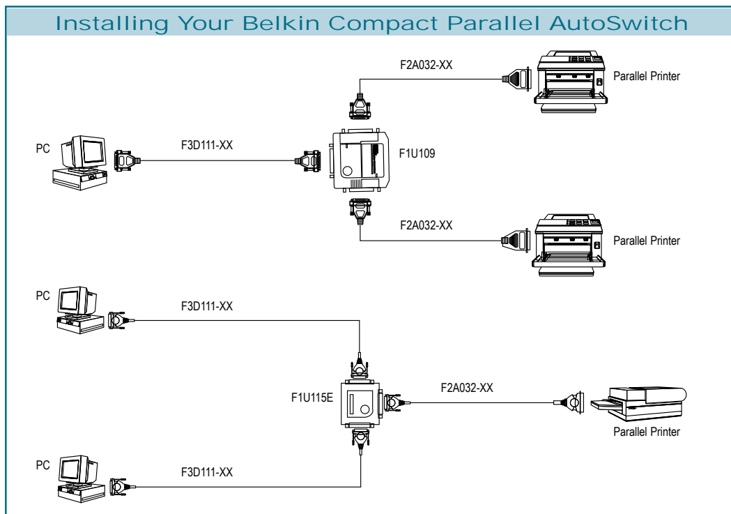
2 Port Reversible AutoSwitch F1U109
